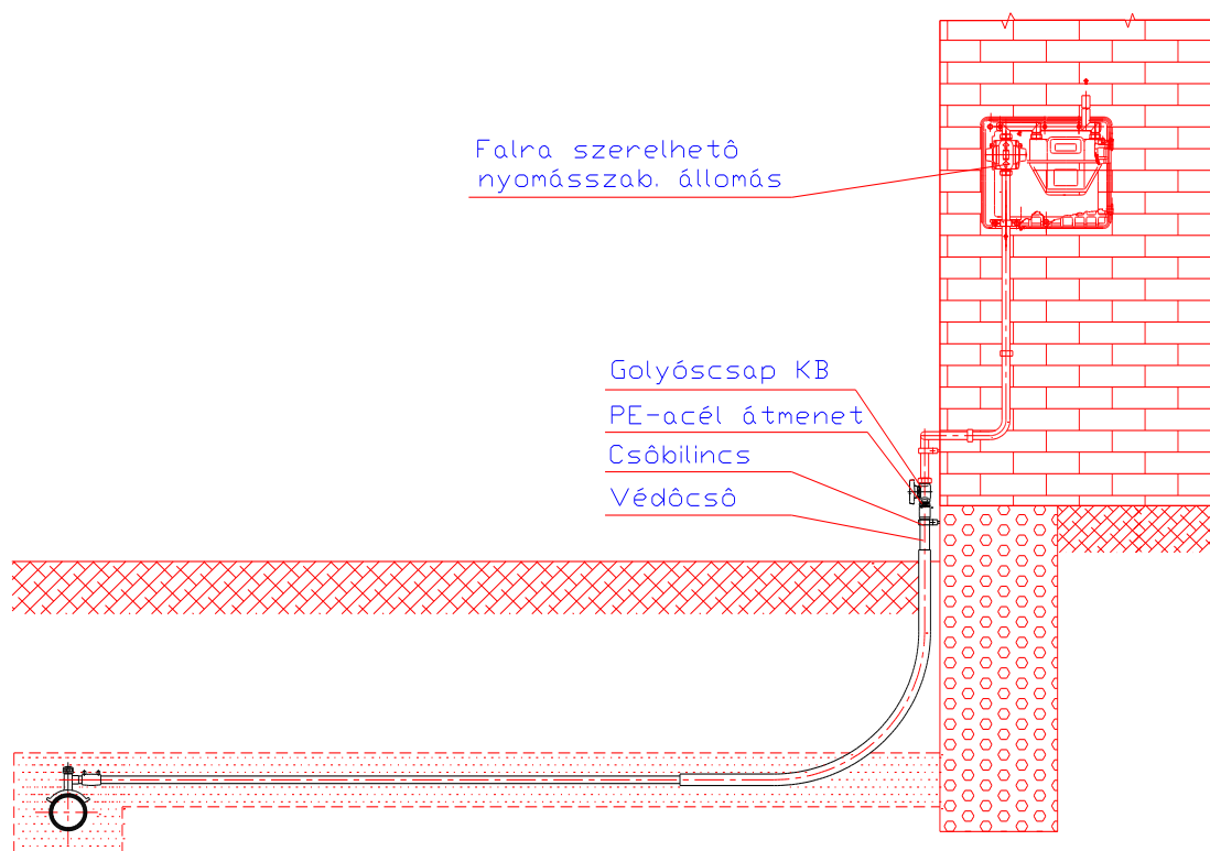
Fali felállás vízszintes vezetékvezetéssel
