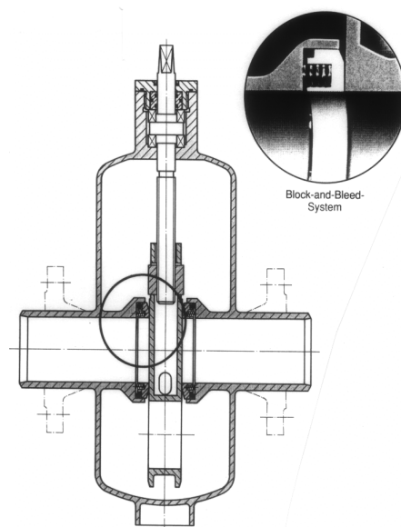
4.4 ábra Nem olajfeltöltésű tolózár DN40-DN300-ig (FRIATEC RHEGA)
