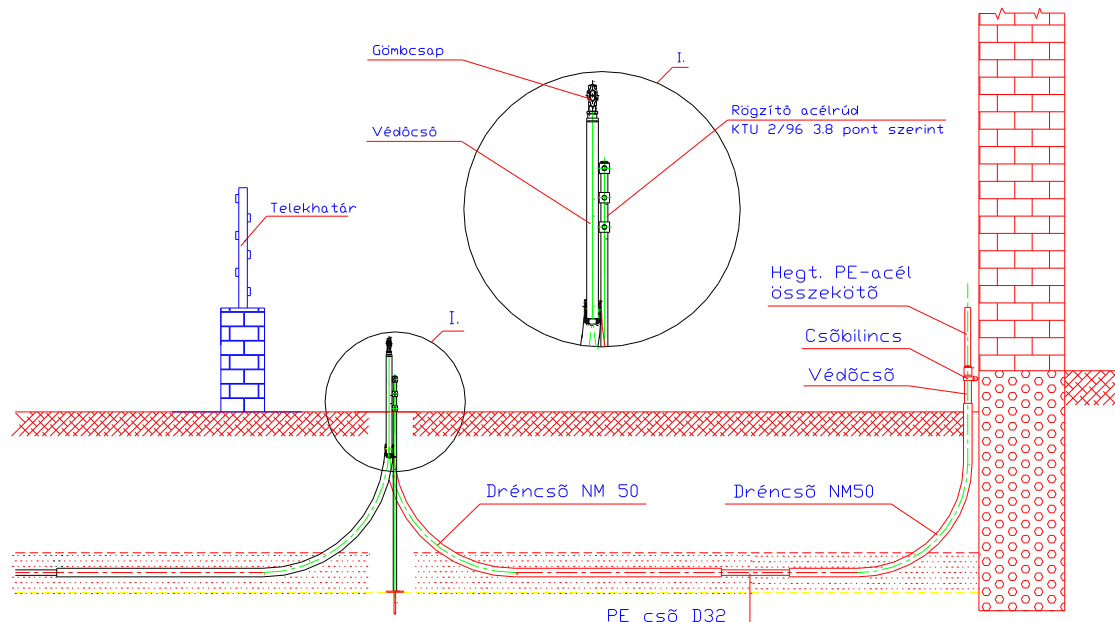
Felállás gömbcsappal acélrúdra/zártszelvényre
