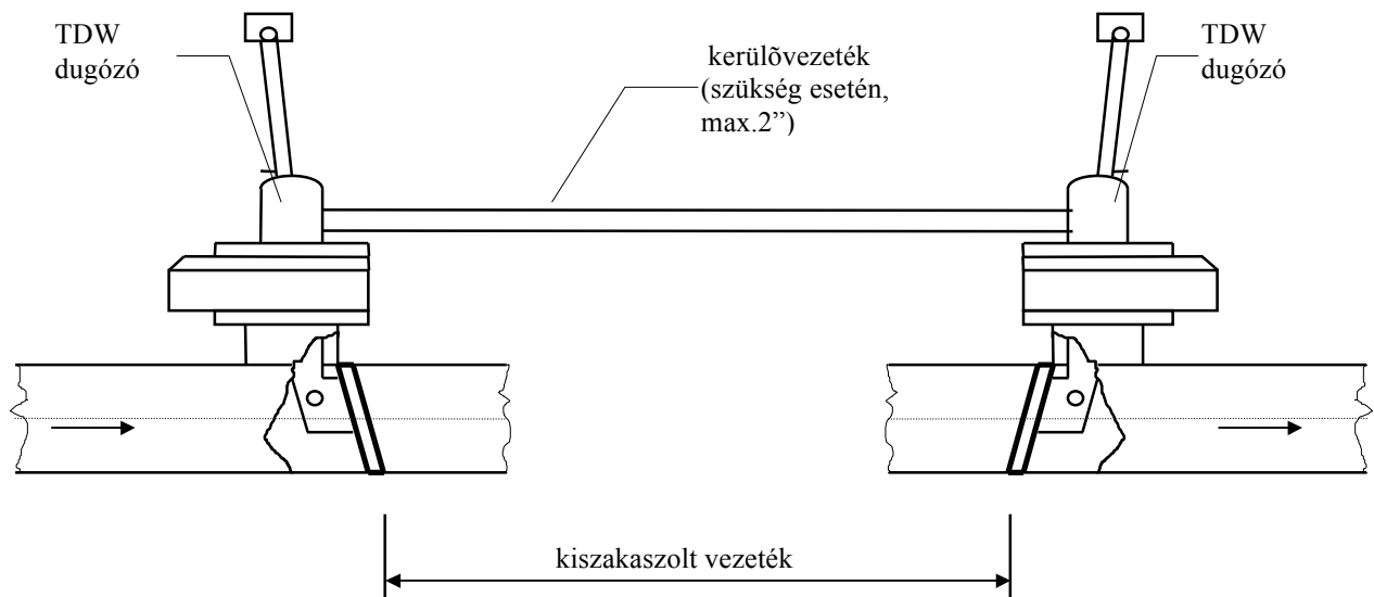
Duplapozíciós kiszakaszolás
