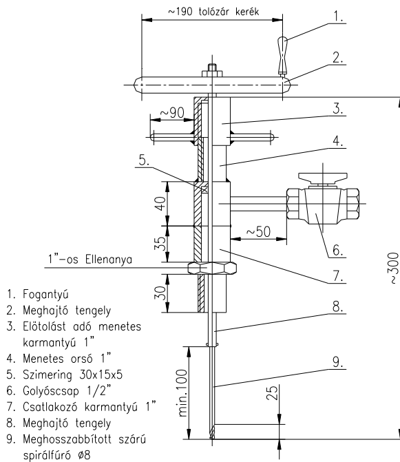
CSÖMEGFŰRŐ SZERELVÉNY
